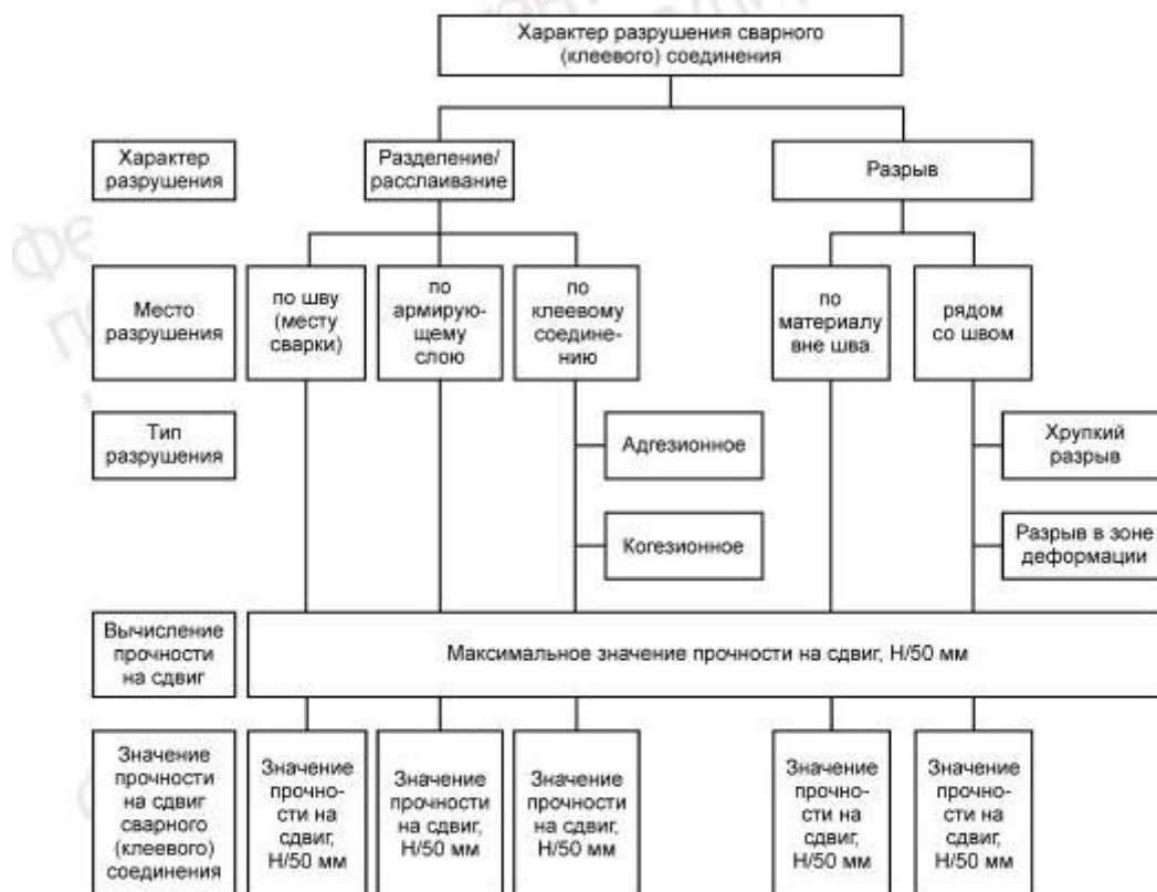
Рисунок А.1 — Характер разрушения сварного (клеевого) соединения
